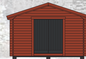
Svergo bod 15 m 2 (3 850x3 850 mm) har ett golv på 25 mm för att klara extra tung belastning. Boden levereras med dubbeldörr samt taksprång. Fönster finns som tillval.
