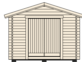
Bruks bod 10 m 2 (3150 x 3150 mm) har ett golv på 25 mm för att klara extra tung belastning. Boden levereras med dubbeldörr. Taksprång 90 cm. Fönster finns som tillval.
