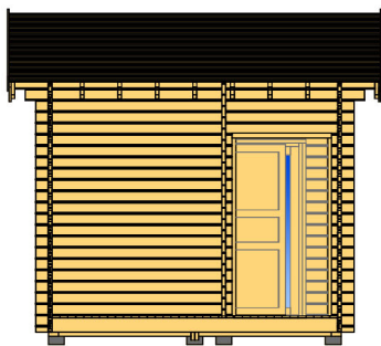
SEKTION A-A
